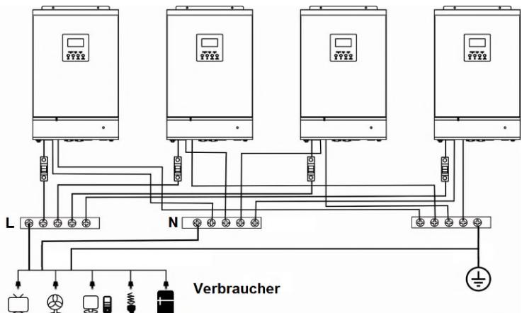
Abb. 5-20 Anschluss der Verbraucher einer einphasigen Parallelanlage.
