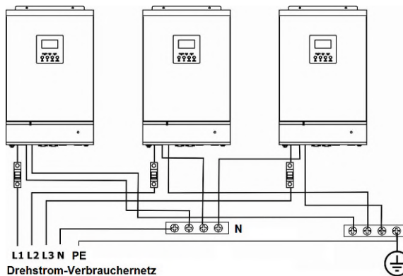
Abb. 5-22 Anschluss der Netz-Versorgung einer einphasigen Parallelanlage.
