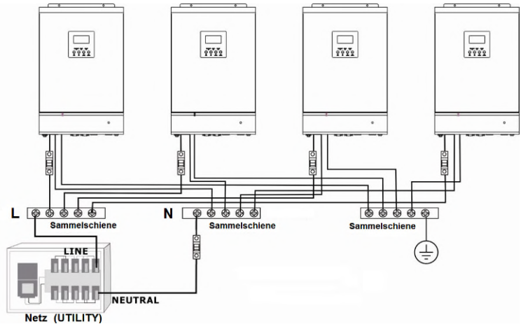
Abb. 5-19 Anschluss der Netz-Versorgung einer einphasigen Parallelanlage.
